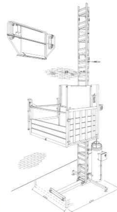
Zur Absturzicherung werden an den Be- und Entladestellen feuerverzinkte Etageeinrichtungen (1 Stück im Lieferumfang enthalten) mit mechanisch verriegelter Schiebetür montiert.
